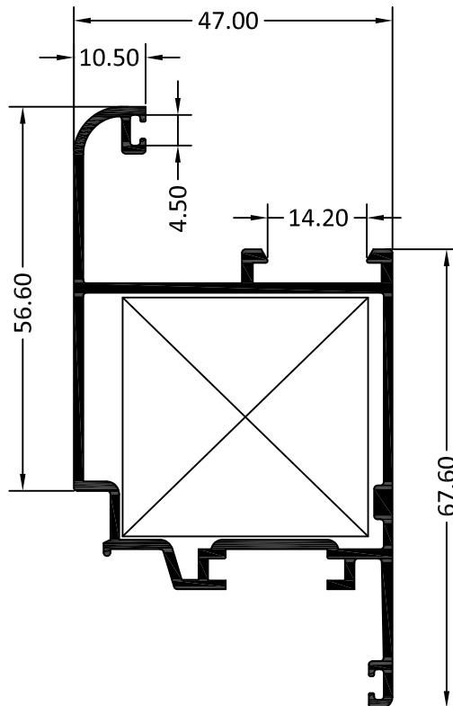
5210 HOJA CERRADA LABI 22
