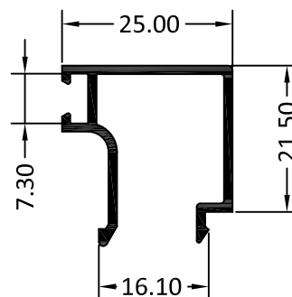
5240 JUNQUILLO HUECO 10
