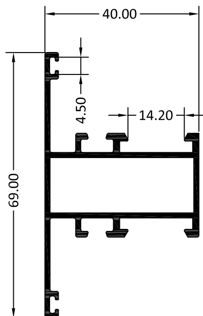
5204 PERFIL "T" PUERTA
