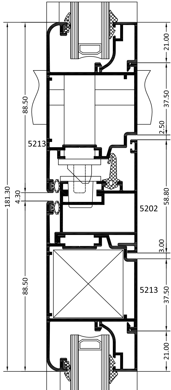
SECCIÓN S14
