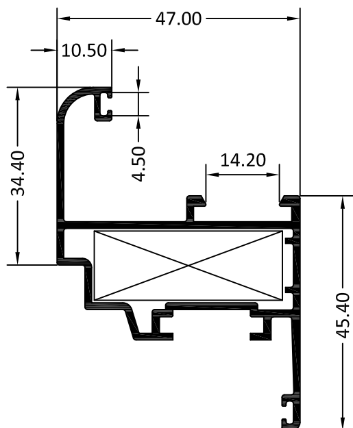
5201 HOJA VENTANA
