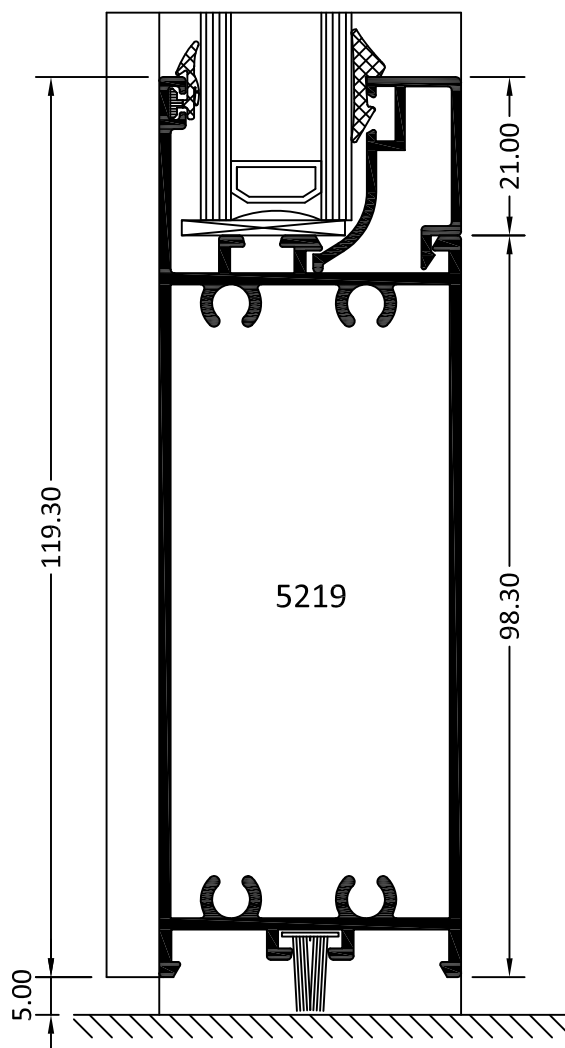
SECCIÓN S11
