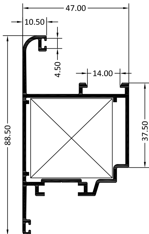
5213 HOJA PUERTA EXTERIOR
