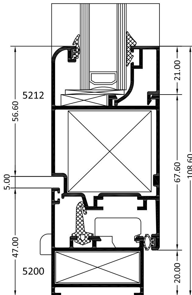
SECCIÓN S7
