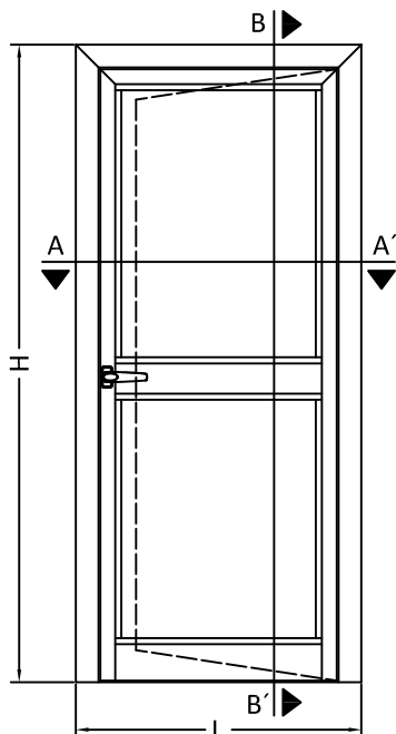
ALZADO
