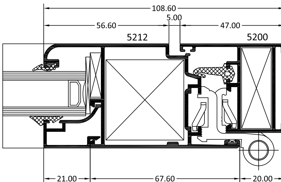
SECCIÓN S10
