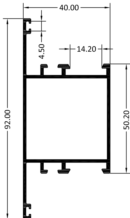
5204 PERFIL "T" PUERTA
