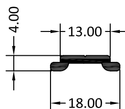
5237 PLETINA ALUMINIO NEGRA
