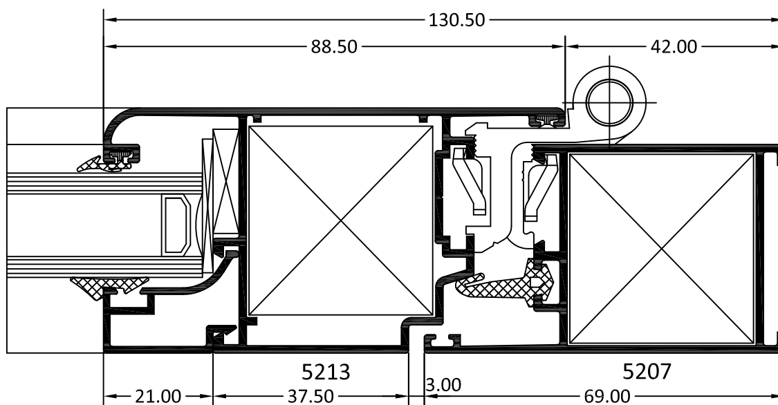
SECCIÓN S15
