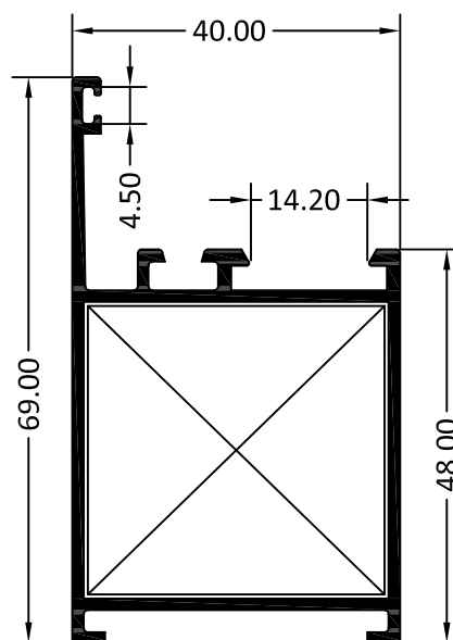
5207 MARCO DE PUERTA
