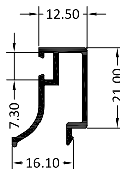
5246 JUNQUILLO HUECO 22
