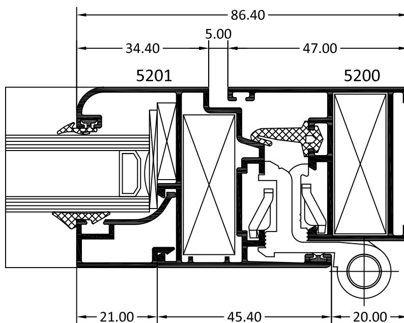
SECCIÓN S4
