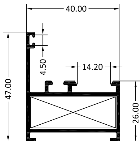
5200 MARCO DE VENTANA
