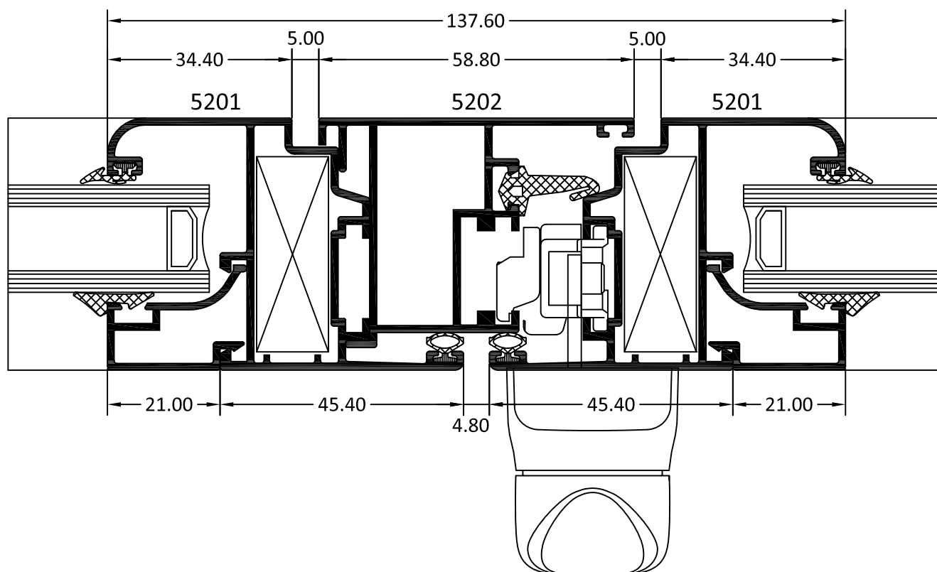
SECCIÓN S3
