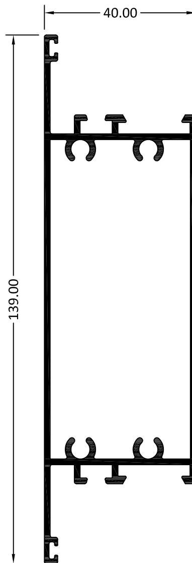
5214 ZÓCALO CENTRAL
