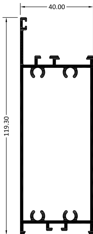
5219 ZÓCALO INFERIOR
