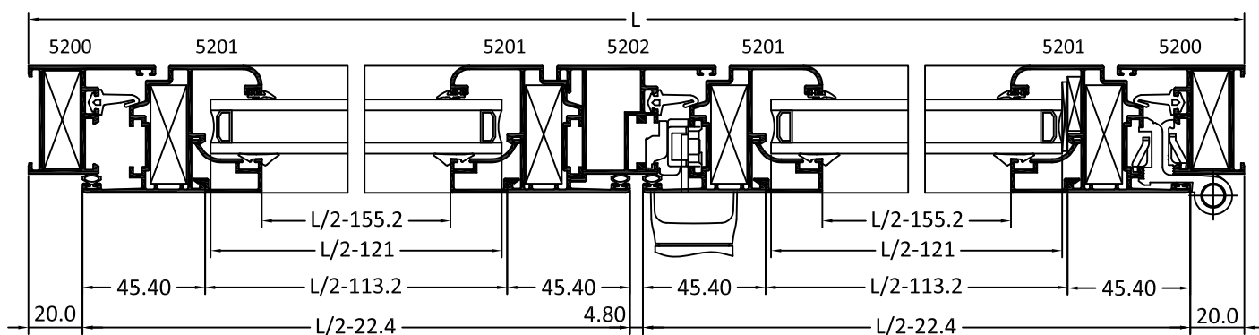
SECCIÓN HORIZONTAL A-A'
