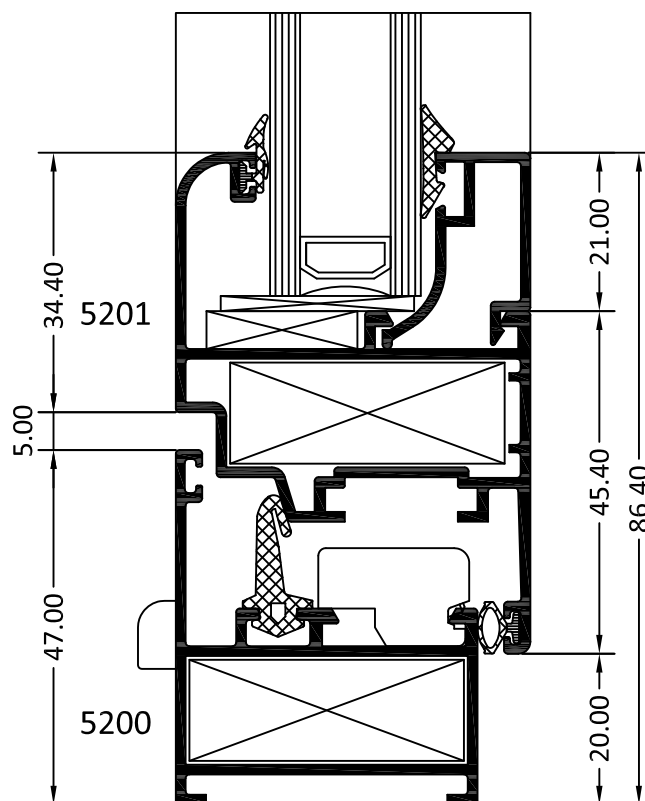
SECCIÓN S1
