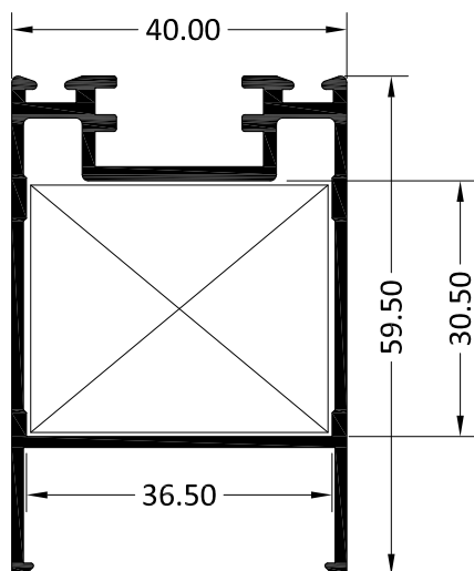
3106 HOJA DE PUERTA MALLORQUINA
