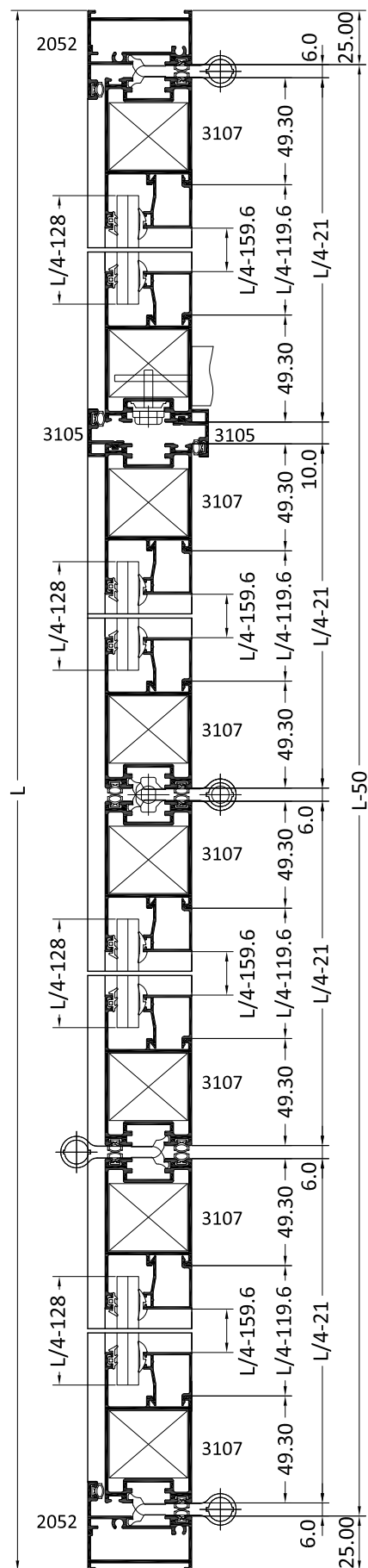
SECCIÓN HORIZONTAL A-A'
