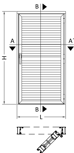
ALZADO
