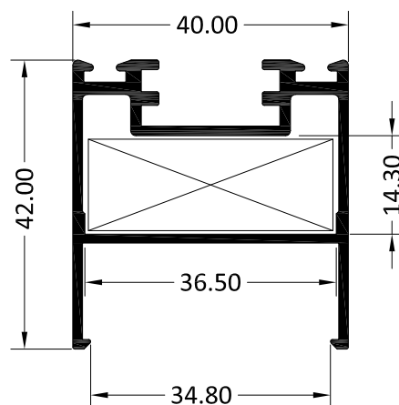
2064 HOJA DE VENTANA MALLORQUINA
