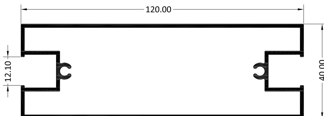
5226 TRAVESAÑO 120 MM MALLORQUINA
