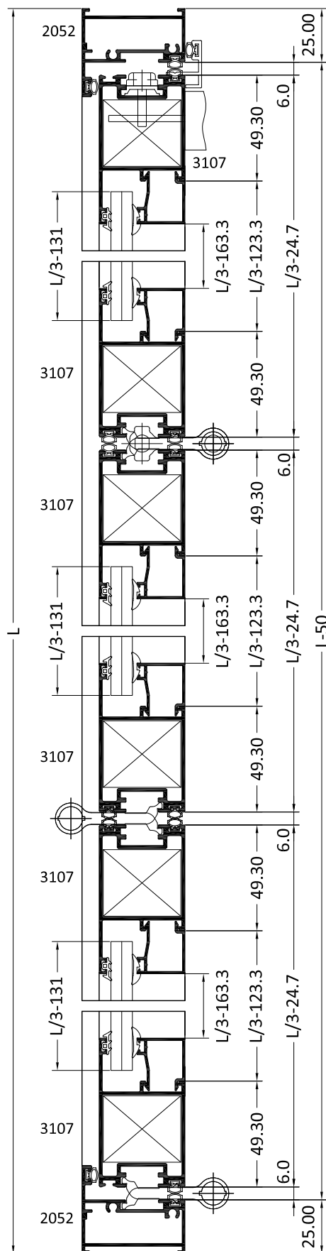
SECCIÓN HORIZONTAL A-A'
