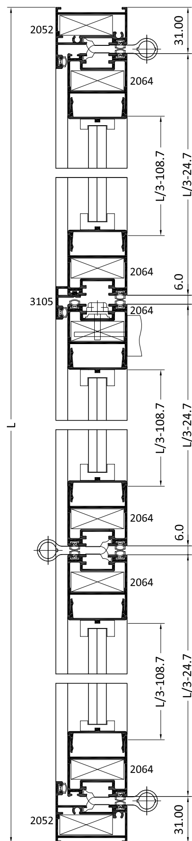
SECCIÓN HORIZONTAL A-A'
