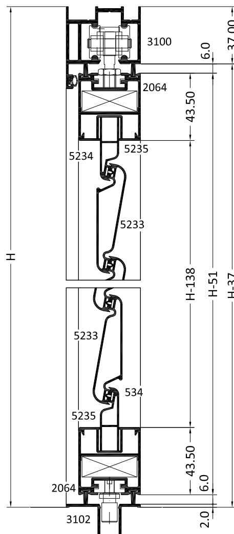
SECCIÓN VERTICAL B-B'
