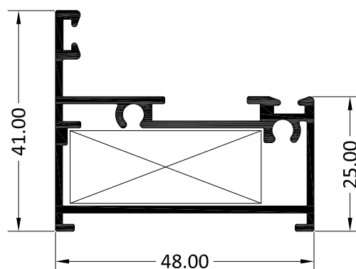
2052 MARCO LATERAL
