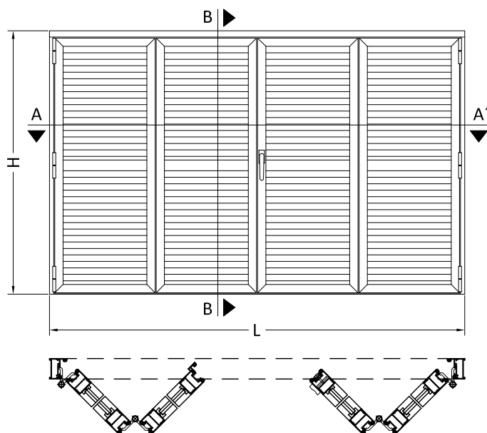
ALZADO
