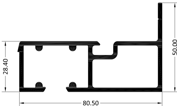
2061 MARCO SUPERIOR CORREDERA
