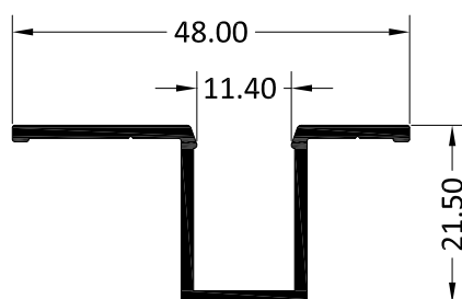
3102 GUÍA INFERIOR EMPOTRADA
