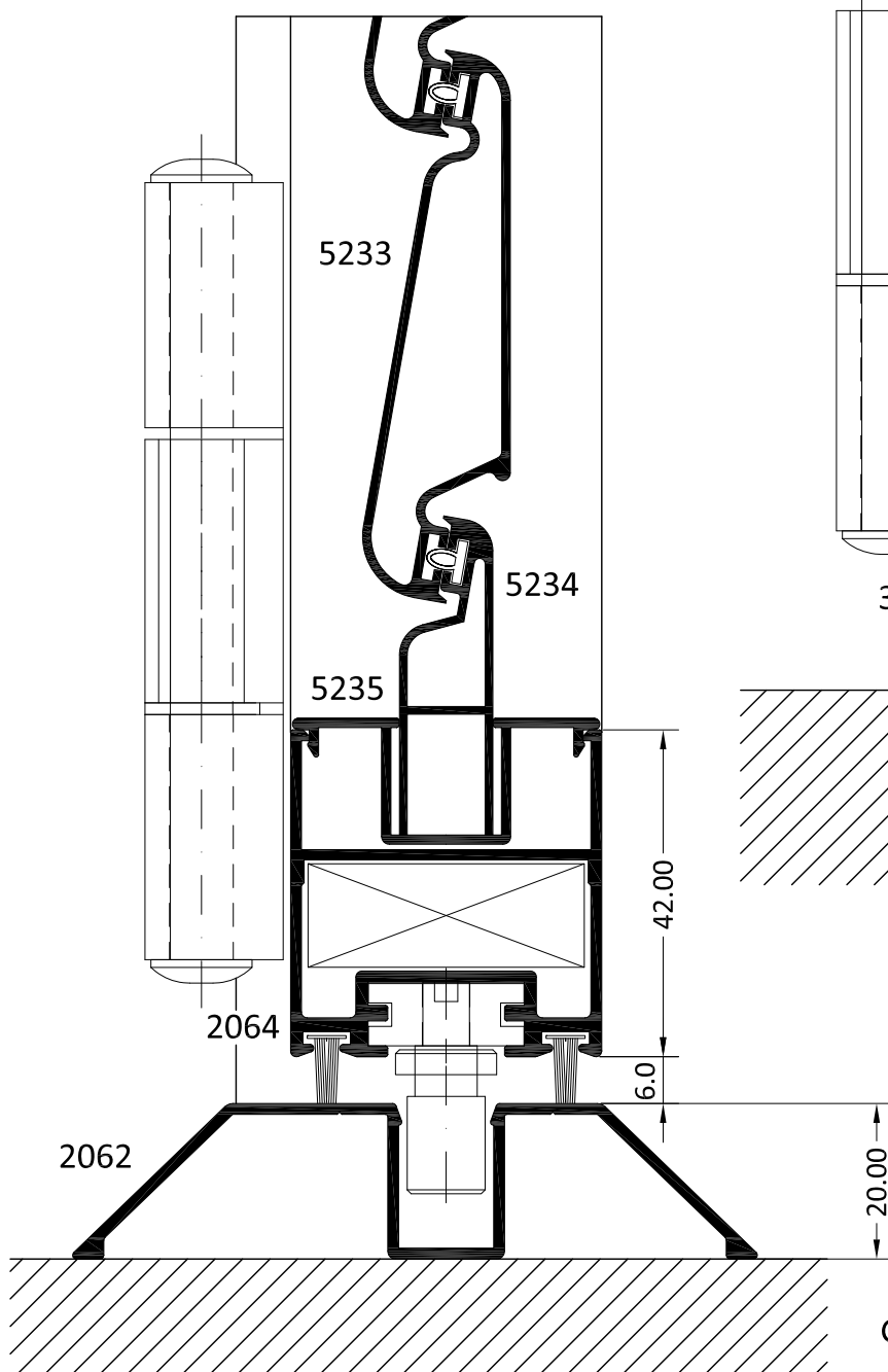
GUÍA INFERIOR EMPOTRADA
