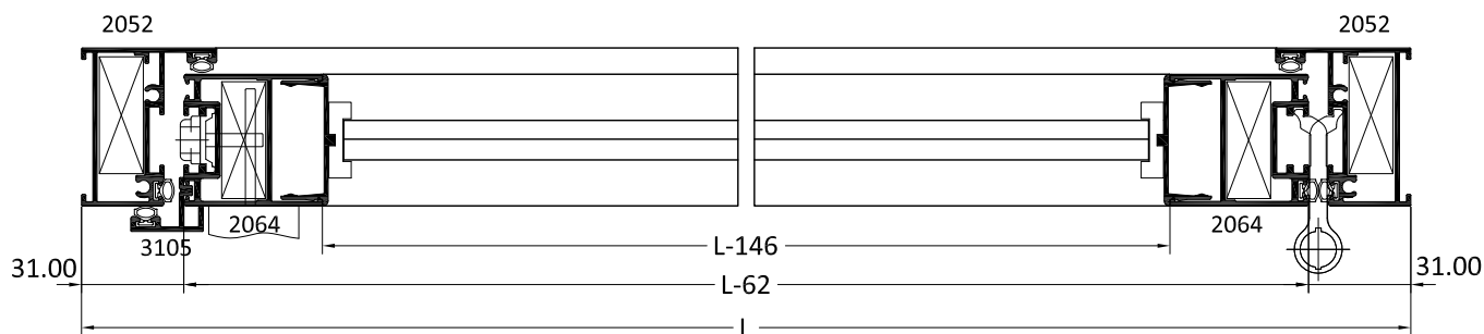
SECCIÓN HORIZONTAL A-A'
