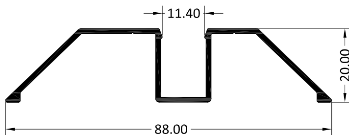
2062 GUÍA INFERIOR SUPERPUESTA
