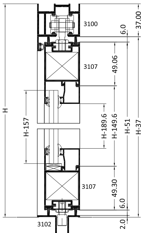
SECCIÓN VERTICAL B-B'
