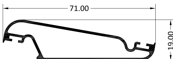
5233 LAMA MÓVIL 71 MM
