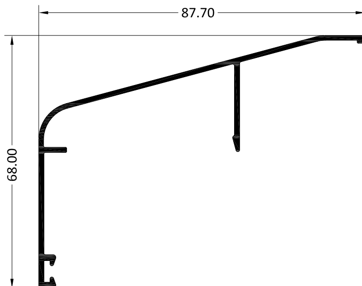
2059 TAPA PARA MARCO SUPERIOR CORREDERA
