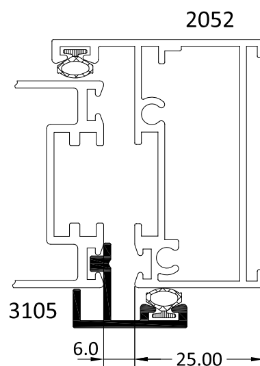
OPCIÓN CIERRE CON PERFIL 3105
