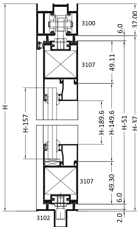
SECCIÓN VERTICAL B-B'
