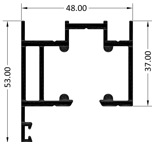
3100 MARCO SUPERIOR
