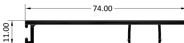
2063 TAPA LATERAL HOJA CORREDERA
