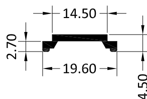
5237 PLETINA CREMONA
