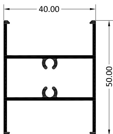
5227 TRAVESAÑO 50 MM MALLORQUINA
